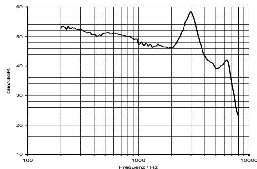
Maximale Verstärkung
