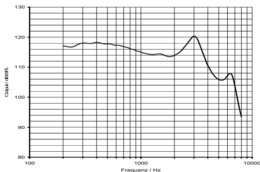
Maximaler Ausgangsschalldruck
